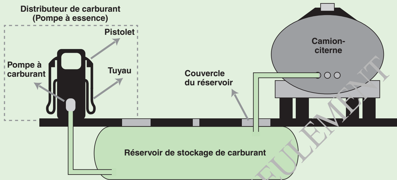
Exemple de processus industriels dans un poste d'essence type
